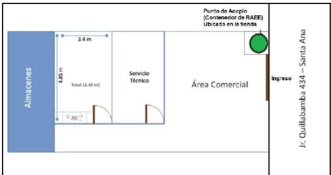
Imagen N° 5: Plano de distribución presentado por el Sistema Colectivo RECYTEC para el punto de acopio MARKEL S.C.R.L.
