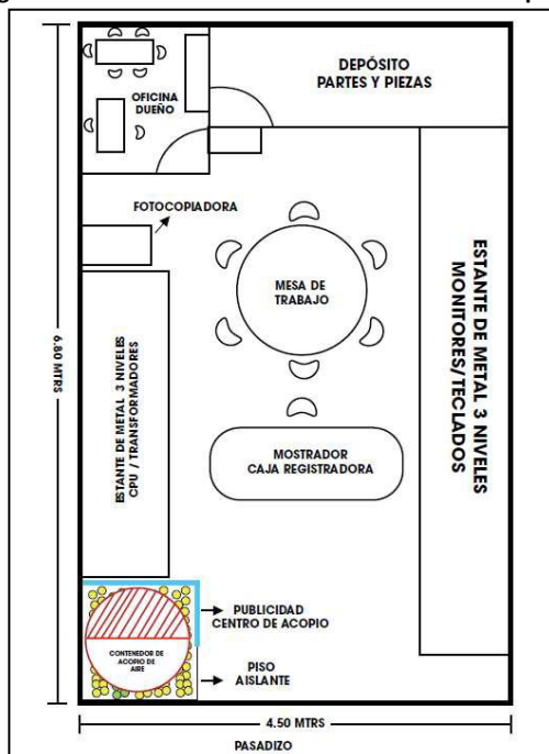
Imagen N° 2: Plano de distribución del Punto de Acopio N°1
