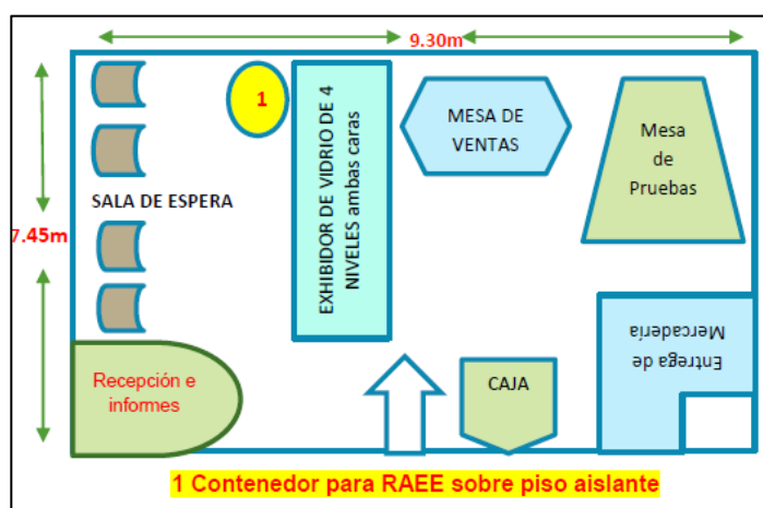
Imagen N° 6: Plano de distribución del punto N° 2.
